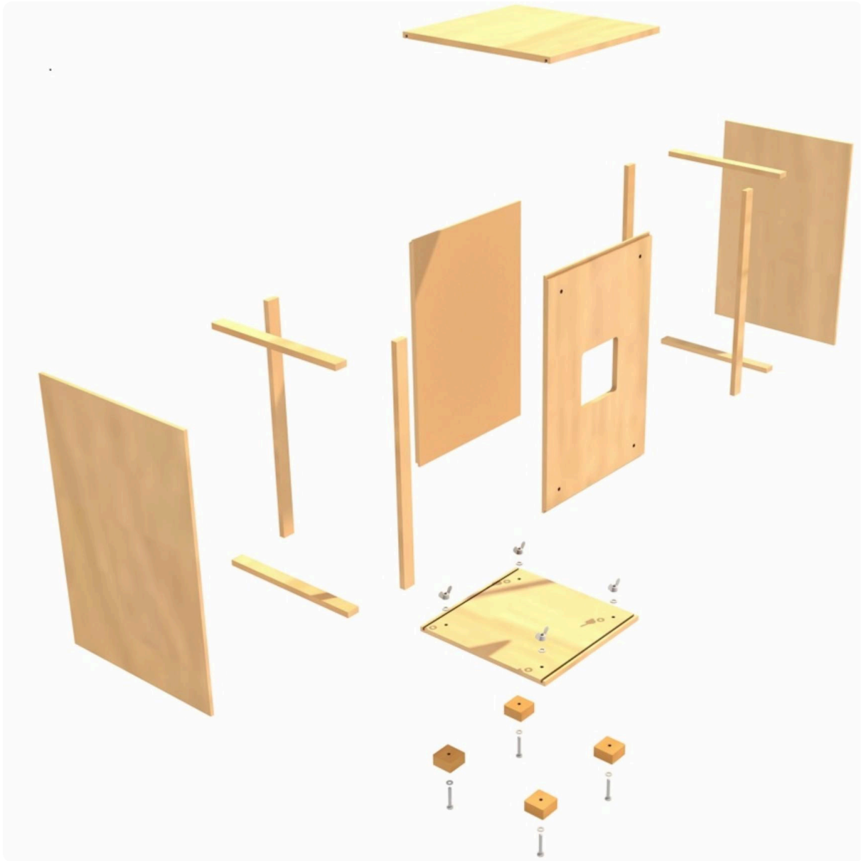
Explosionsbild Cajon
