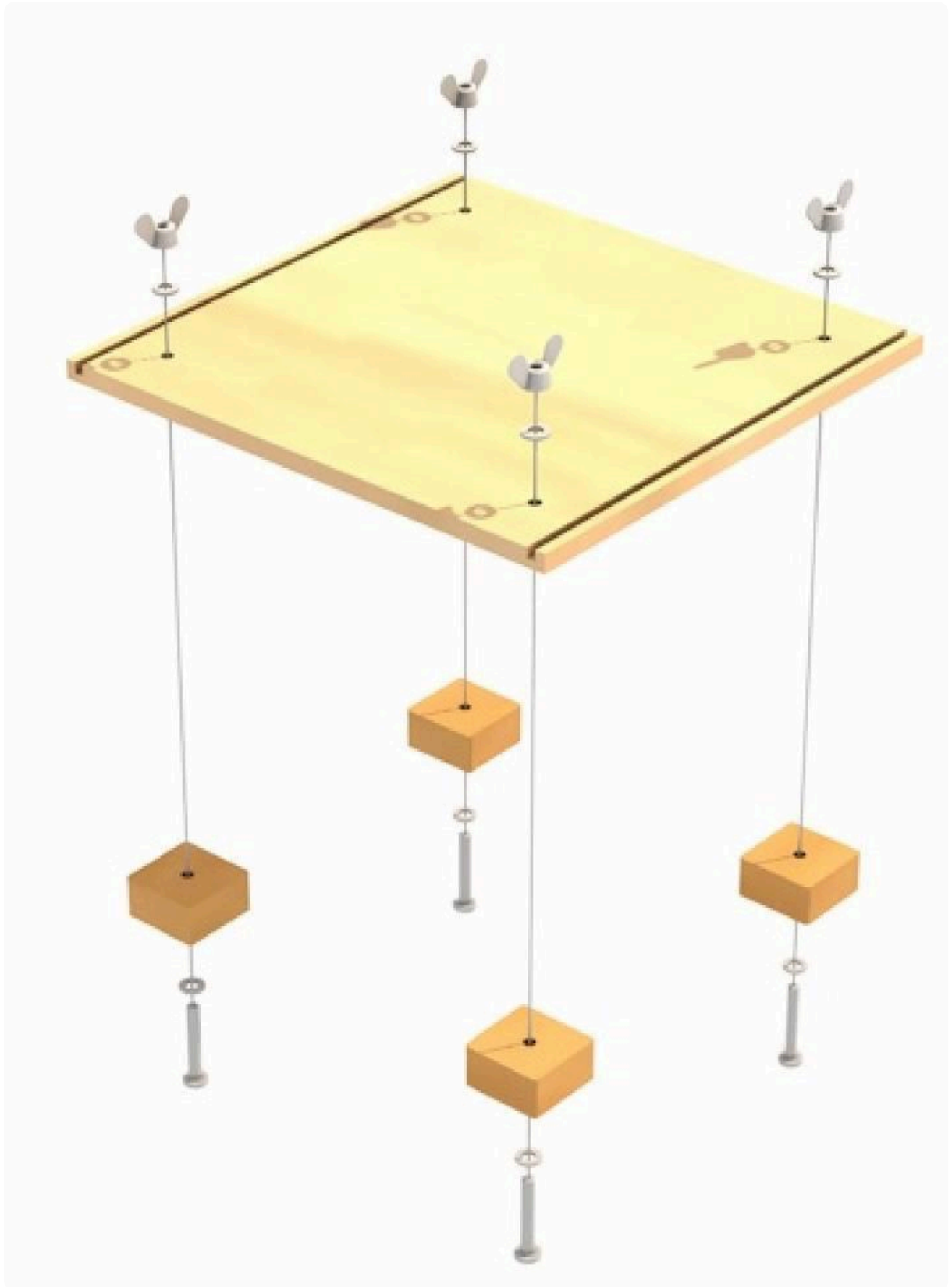
Montage Boden
