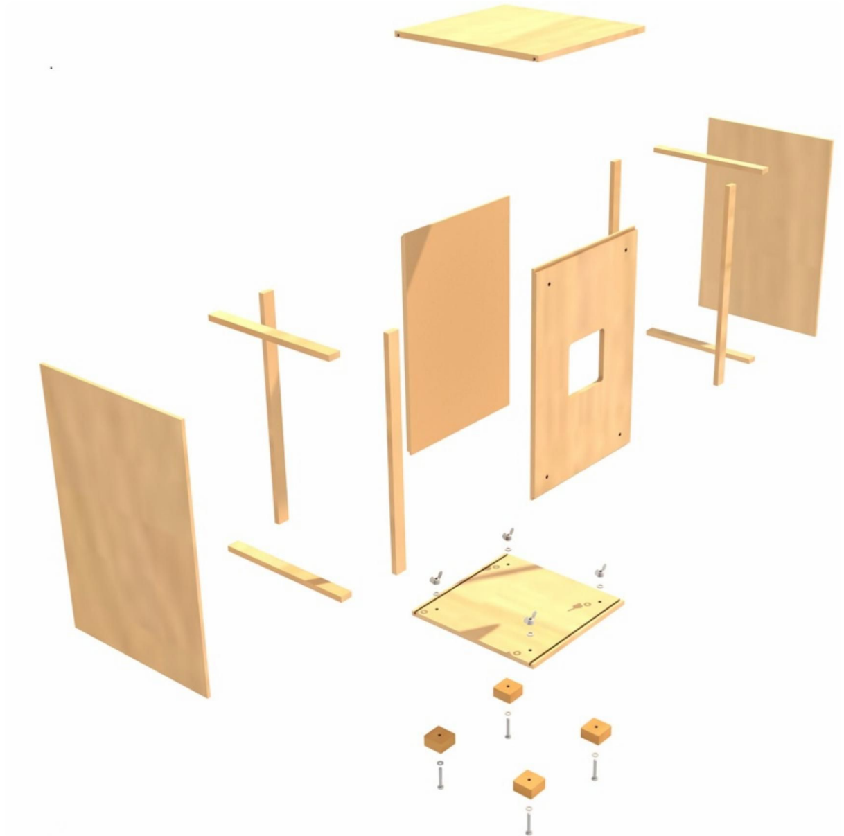
Explosionsbild Cajon
