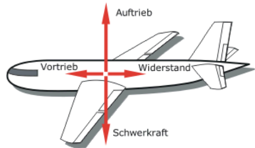
Kraeftegleichgewicht-Flugzeug
