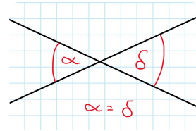
Scheitelwinkelsatz
