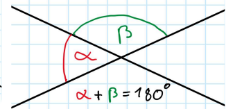
Nebenwinkelsatz
