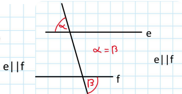
Wechselwinkelsatz
