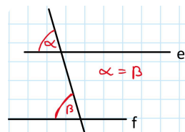
Stufenwinkelsatz
