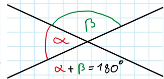
Nebenwinkelsatz
