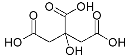
Zitronensäure - Skelettschreibweise
