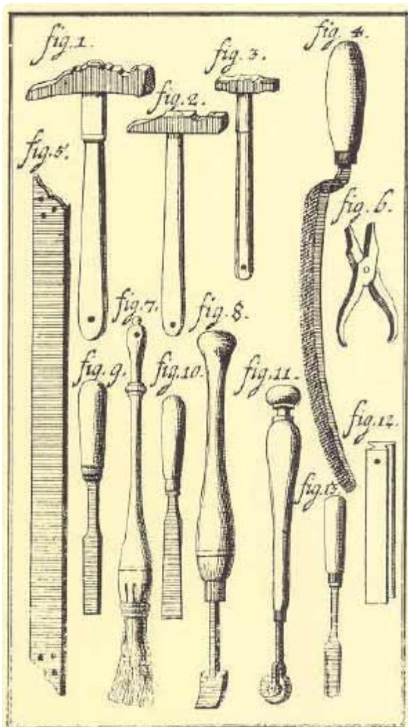
1 Rückenrunde-Hammer – 2 Hammer zum Ableimen – 3 Hämmerlein zum Klausuren-anslagen – 4 Goldschnittraspel – 5 Eisenlineal – 6 Biegezange – 7 Kleisterpinsel – 8 Glättelkolben – 9 Stechbeitel – 10 Stemmeisen – 11 Gravierte Rolle für gepunzte Goldschnitte – 12 Einreibehölzchen für Bünde (Vorläufer der Bünde- zange) – 13 Ecken- abstoßeisen.
