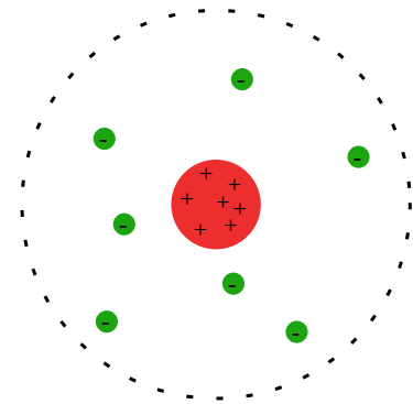
Atommodell nach Rutherford
