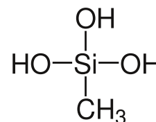
Methylsilantriol
