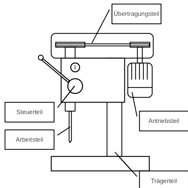
Bohrmaschine
