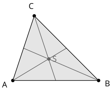
Seitenhalbierende s_a, s_b, s_c und Schwerpunkt S
