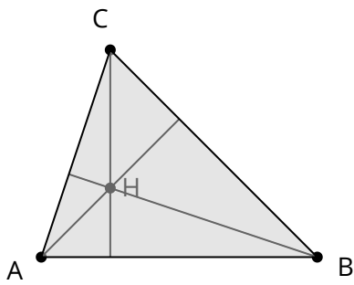
Höhen h_a, h_b, h_c und Höhenschnittpunkt H
