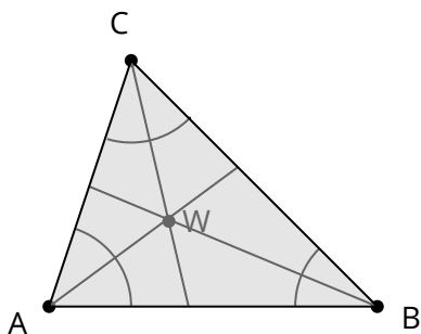
Winkelhalbierende w_a, w_b, w_c und Schnittpunkt W
