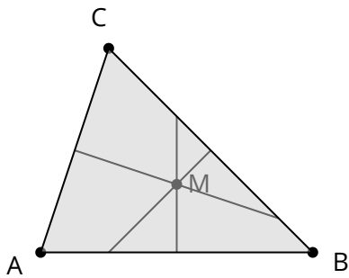
Mittelsenkrechten m_a, m_b, m_c und Schnittpunkt M
