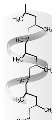
Helix-Polypropylen
