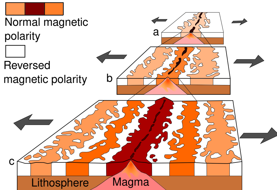
Sea-floor-spreading: Nachweis durch die magnetische Polarität des Meeresbodens
