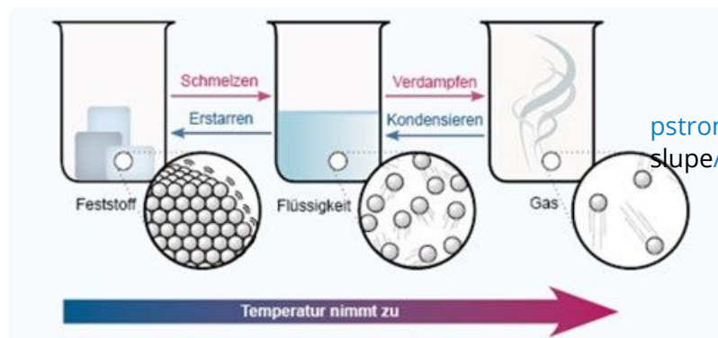
Abbildung 1: Die Teilchenebene
