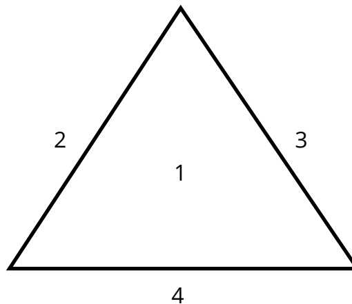
Das Frankfurt-Dreieck:
