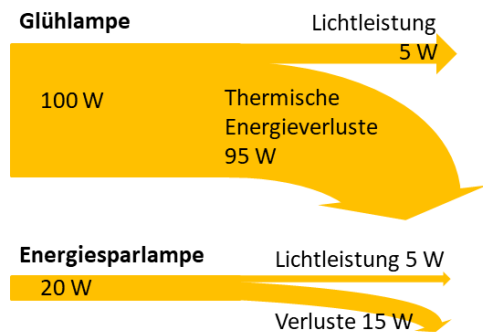
Abb. 1 — Wirkungsgrad einer Glühlampe und einer Energiesparlampe
