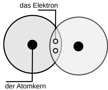
Schalen-Modell eines Wasserstoff-Moleküls
