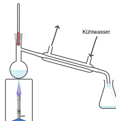
Apparatur 3: Mit Glasrohren und Liebigkühler
