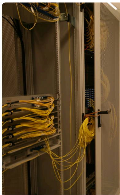
weiterer ServerSwitch-Schrank
