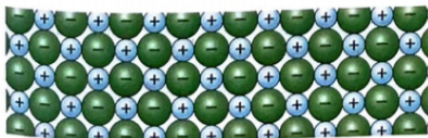
[6] Ionengitter
