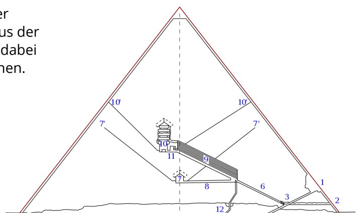
Querschnitt der Cheopspyramide
