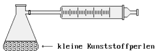
Aufbau zum Ermitteln der molaren Masse
