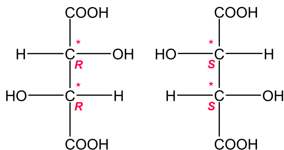
Abb. 1 — Chiralität visualisiert
