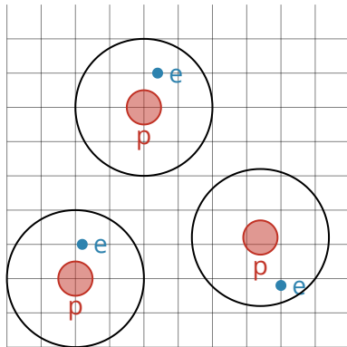
Normale Atome
