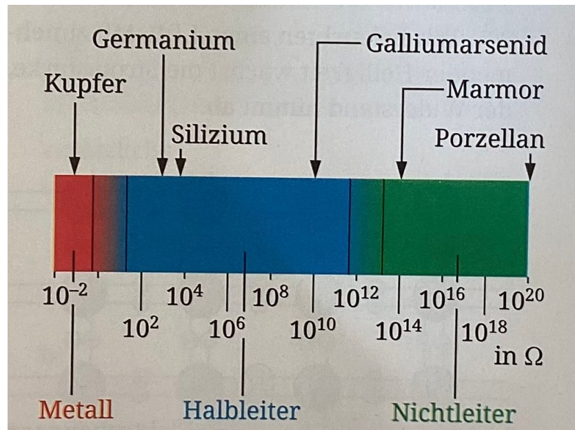
Widerstand von Leiter - Halbleiter - und Nichtleiter bei Raumtemperatur
