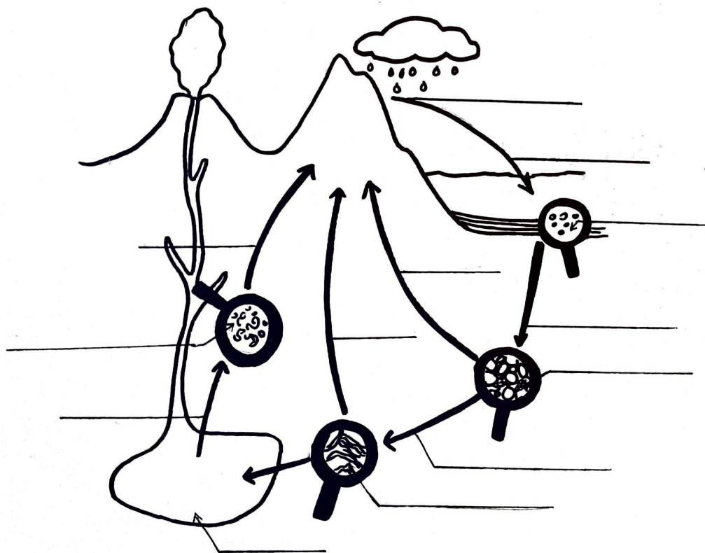
Der Gesteinskreislauf
