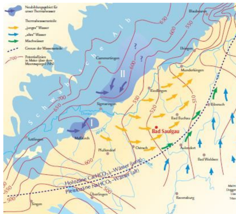
Fließrichtung des unterirdischen Wassers
