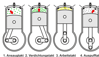
1. Ansaugtakt 2. Verdichtungstakt 3. Arbeitstakt 4. Auspufftakt
