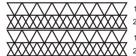
Abb. 2: Zweischichtmineral
