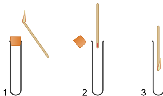
Durchführung: Glimmspanprobe
