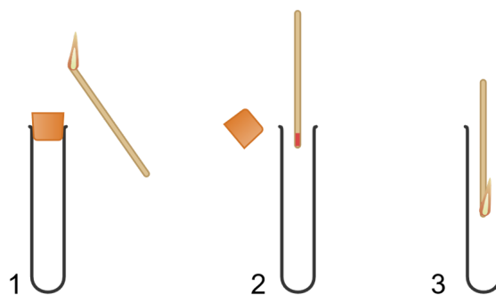
Durchführung: Glimmspanprobe
