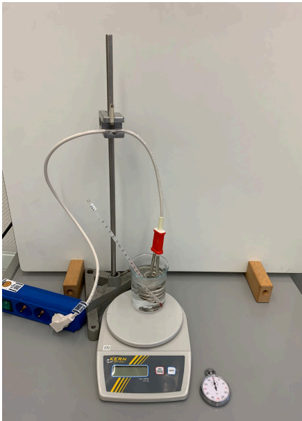
Versuchsaufbau
