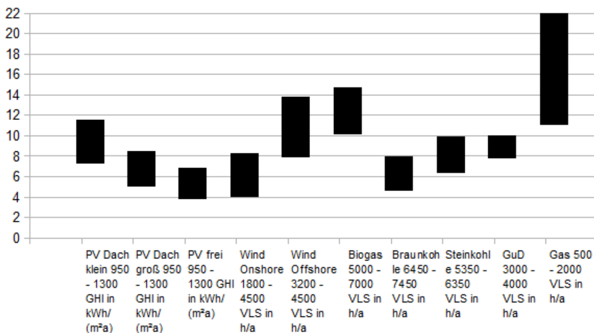
Abb. 2 — Stromgestehungskosten (€cent pro kWh)
