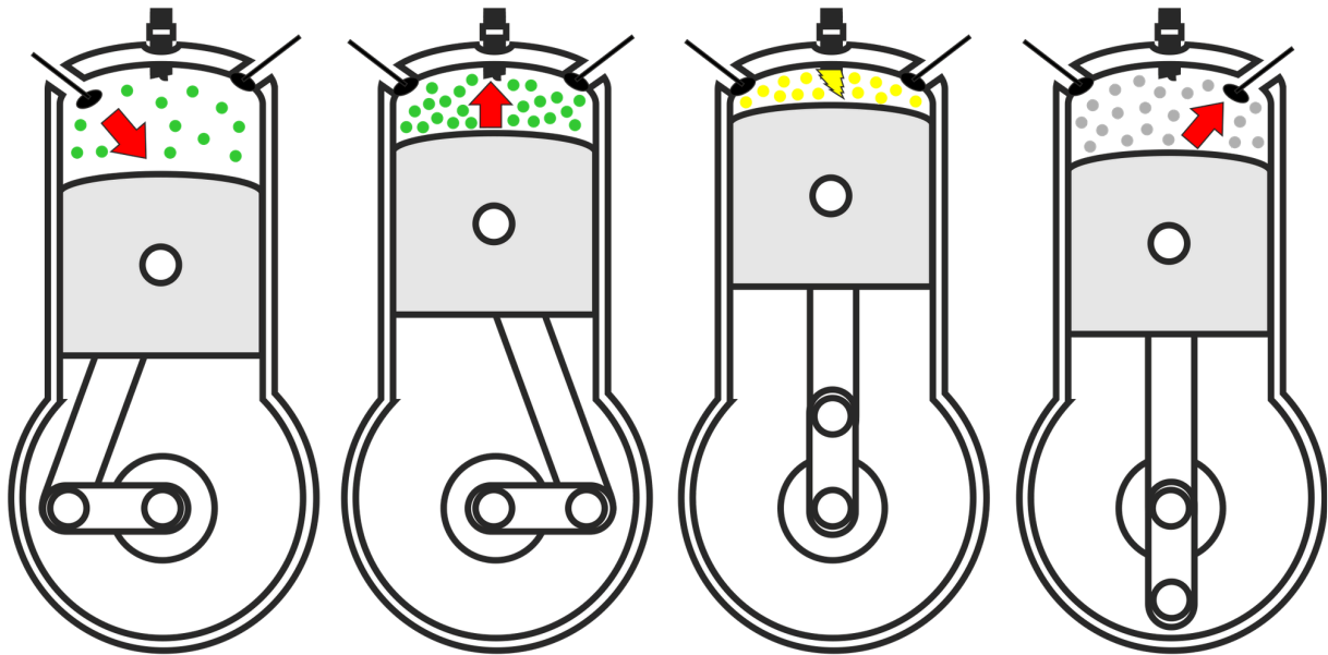
1. Ansaugtakt 2. Verdichtungstakt 3. Arbeitstakt 4. Auspufftakt
