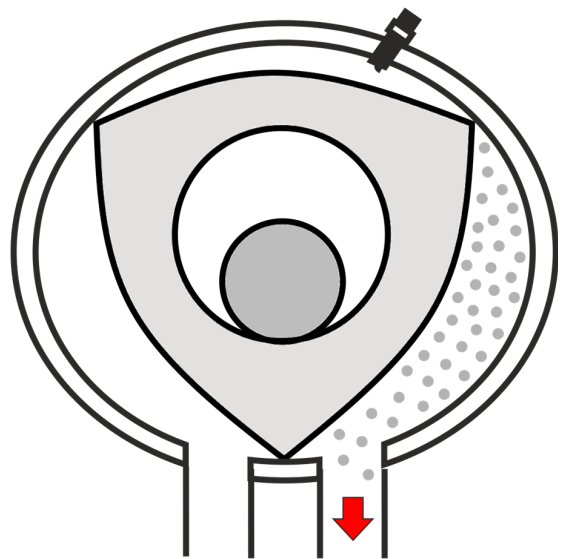
4. Auspufftakt
