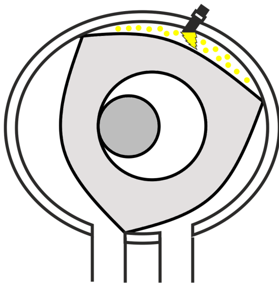
3. Arbeitstakt
