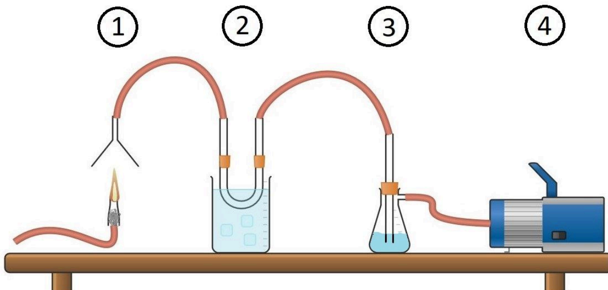
Abbildung 1 - Apparatur zum Nachweis der Verbrennungsprodukte von Wasserstoff.
