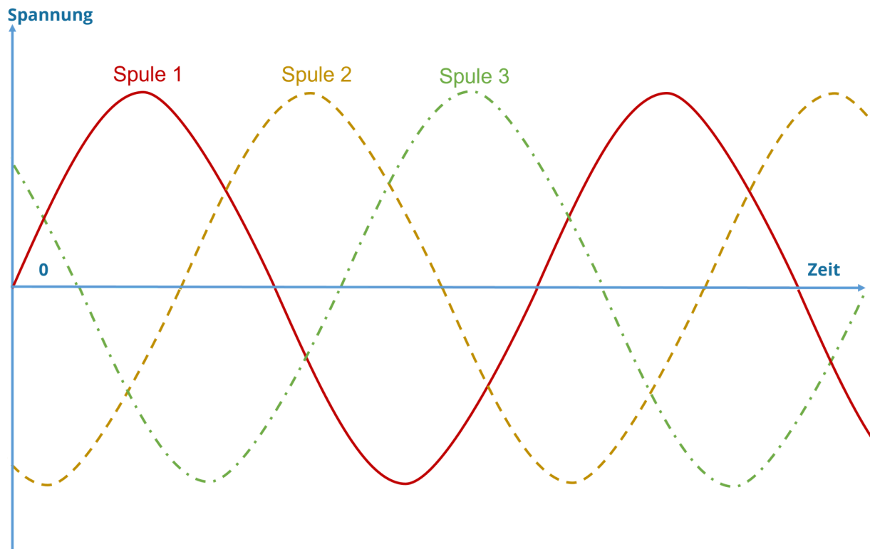
Drehstromsystem mit 3 Spulen
